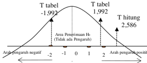
Gambar 2: Kurva Regresi Linear X_2 - Y
