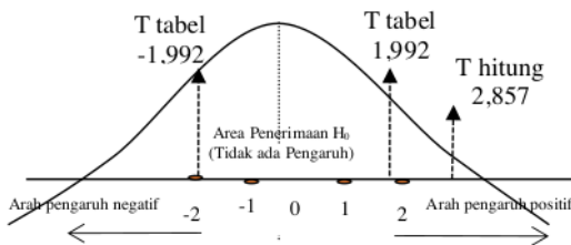
Gambar 1 : Kurva Regresi Linear X_1 - Y
